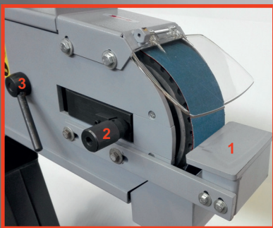
1-squadro supporto pezzo 2-dispositivo centratura nastro 3-leva cambio rapido del nastro
