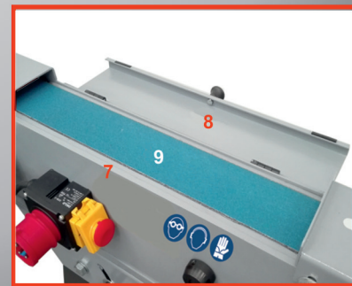
7-piano di lavoro mm 460x100 8-protezione mobile: massima sicurezza 9-nastro abrasivo allo Zirconio gr.60
