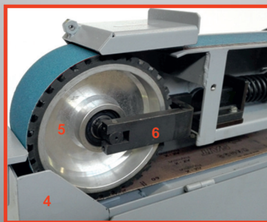
4-scatola raccolta trucioli amovibile 5-puleggia gommata di trascinamento 6-robusto sistema di tensione del nastro
